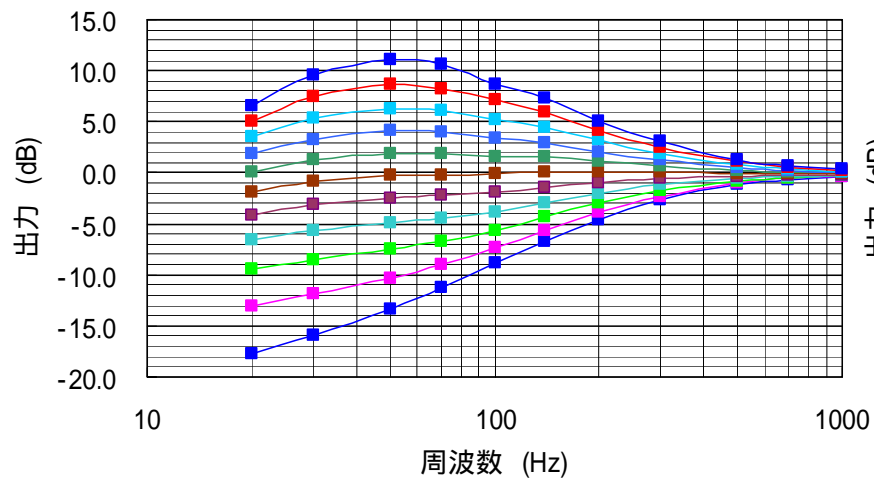
低域トーンコントロール特性( f_c=300\text{Hz} )
