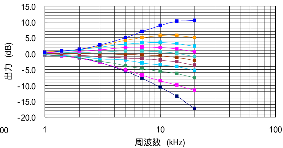
高域トーンコントロール特性( f_c=6\text{kHz} )
