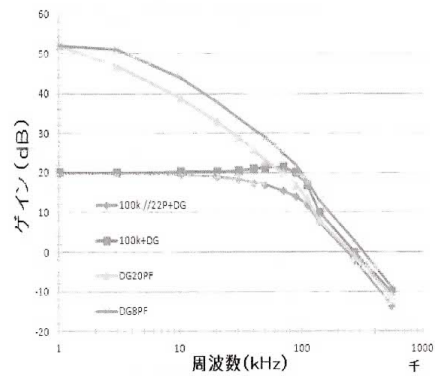
A 級 OPT付き2段増幅FETシングルアンプ
