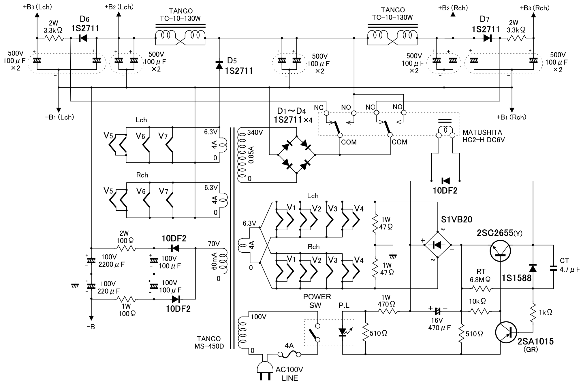
[ 図9 ] 電源回路
