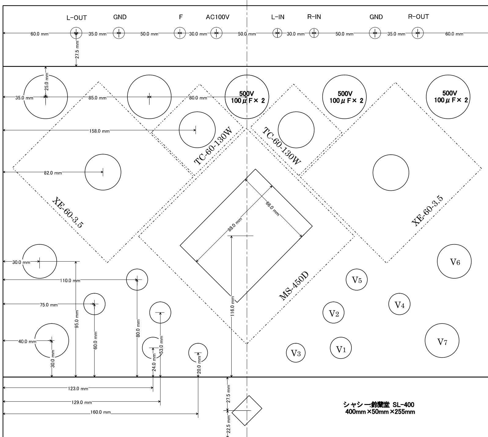
[ 図10 ] シャシ - 部品配置
