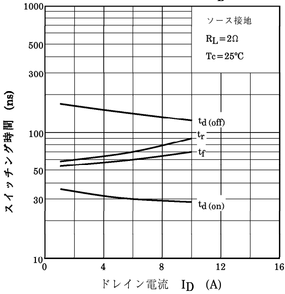
スイッチング時間 - I_D
