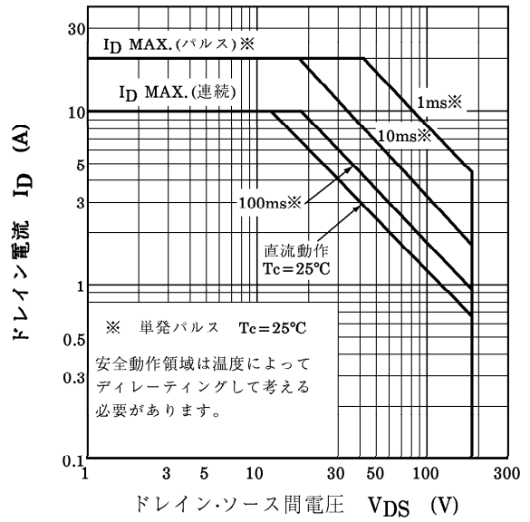
安全動作領域
