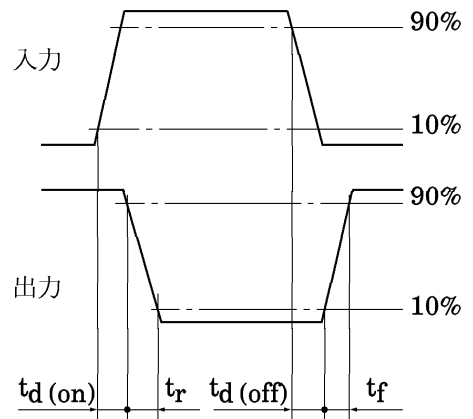
応答波形
