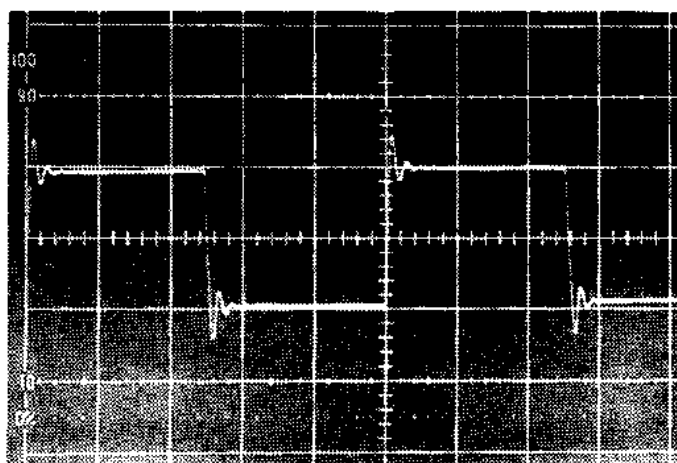
[写真 6] 10kHz 方波形 V軸：2V/DIV 負荷： 8\Omega // 0.1\mu\text{F}
