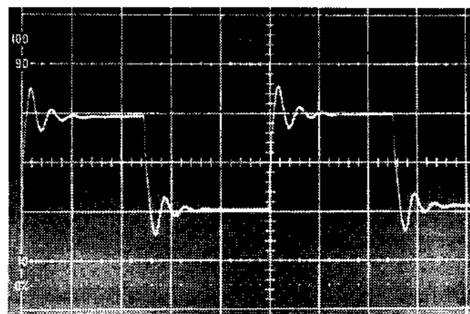
[写真 7] 10kHz 方波形 V軸：2V/DIV 負荷： 8\Omega // 0.47\mu\text{F}
