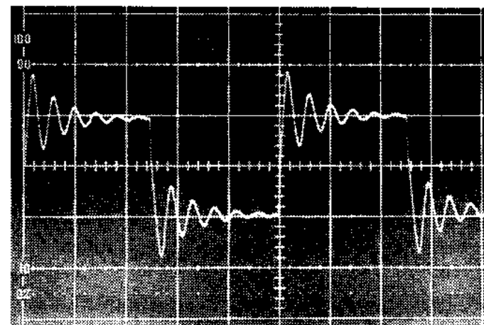
[写真 4] 10kHz 方波形 V軸：2V/DIV 負荷： 0.47\mu\text{F}
