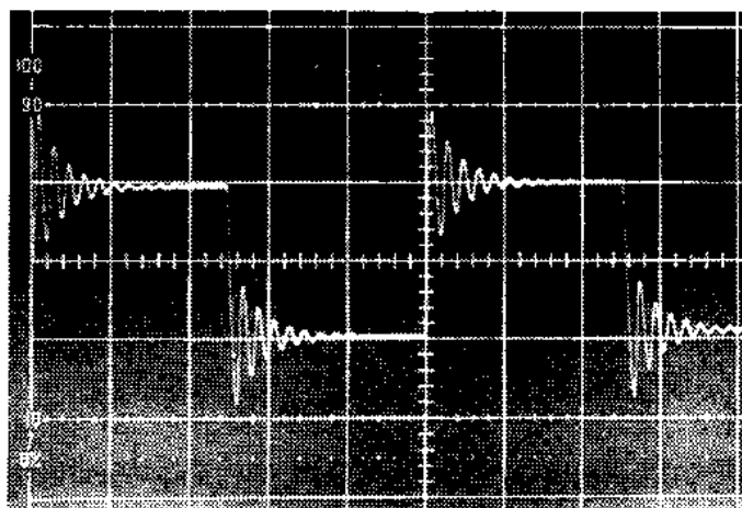
[写真 3] 10kHz 方波形 V軸：2V/DIV 負荷： 0.1\mu\text{F}
