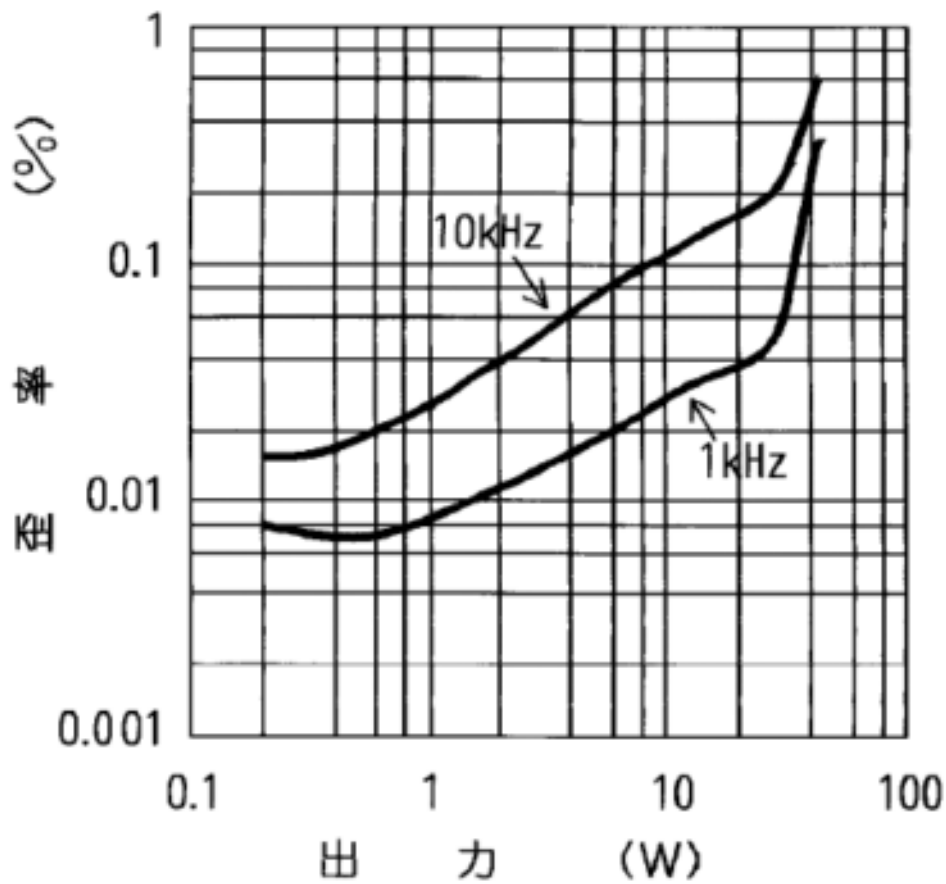
歪み率特性
