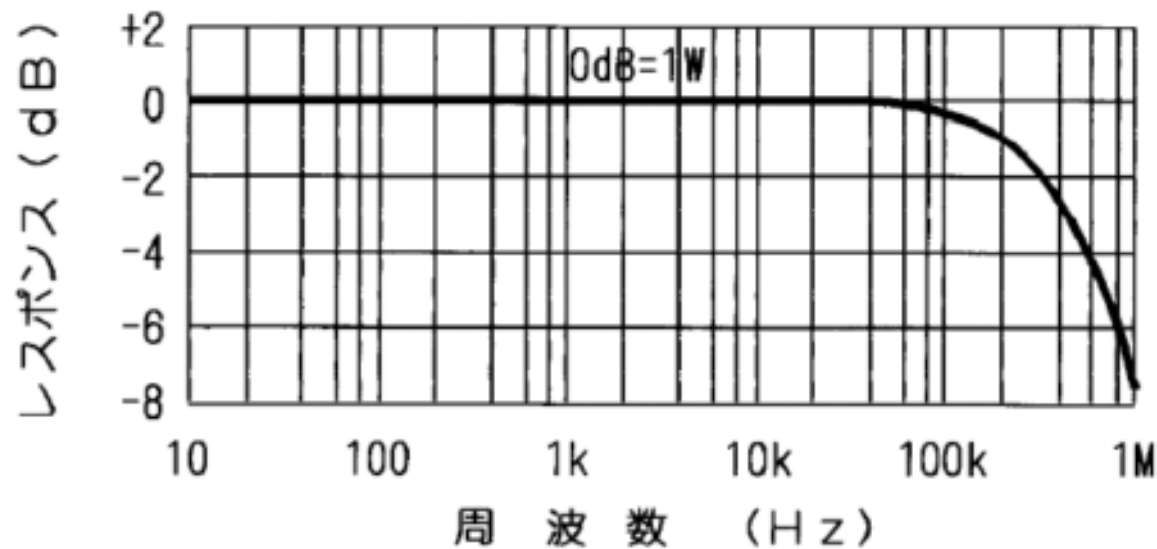
周波数特性
