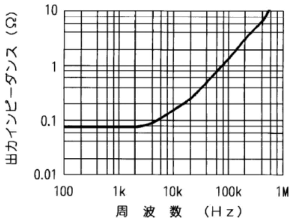
出力インピーダンス特性
