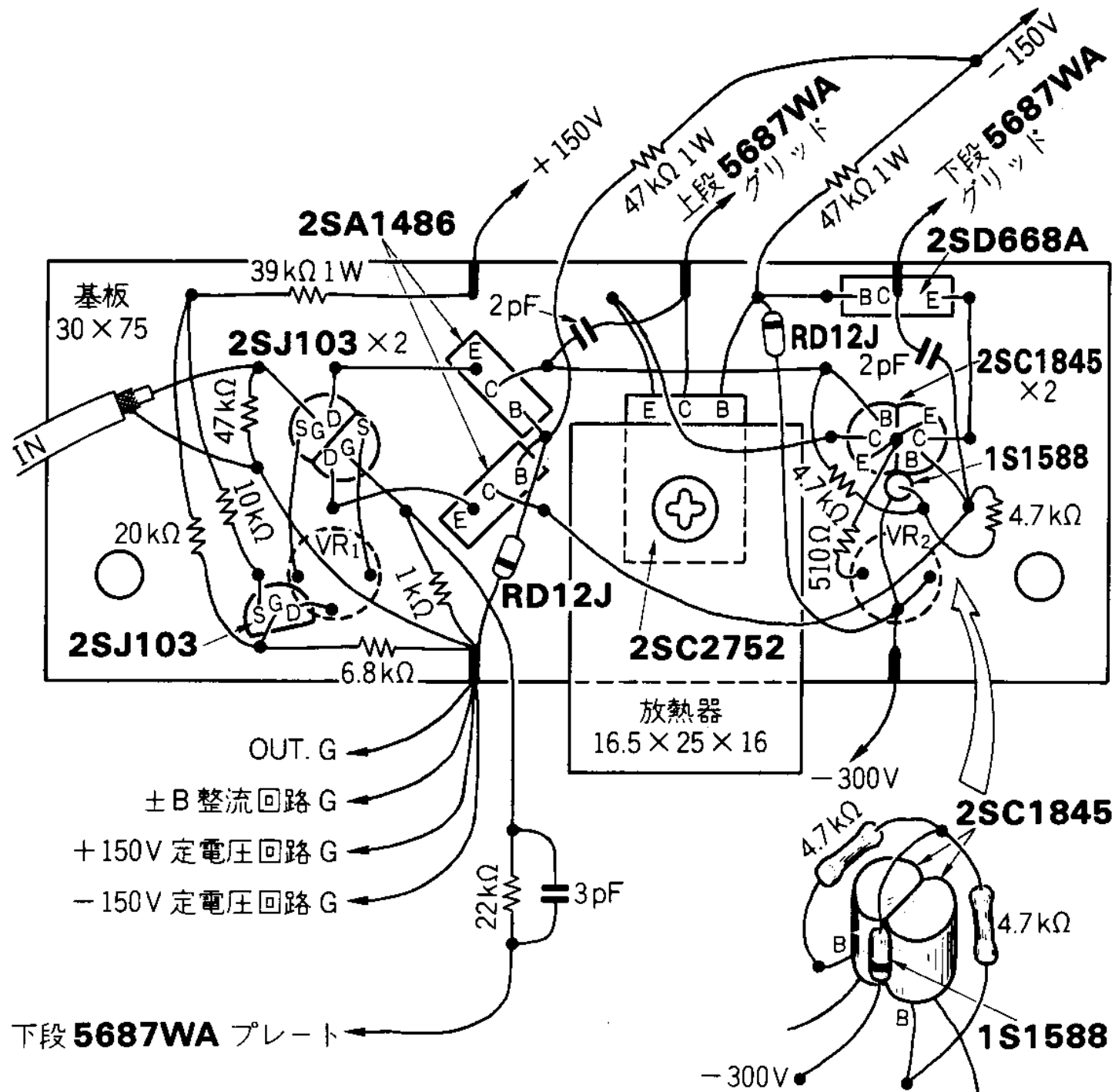
[図17] アンプ回路基板の配線 (部品取り付け面より見る。VR 1 , VR 2 は裏側に取り付け)
