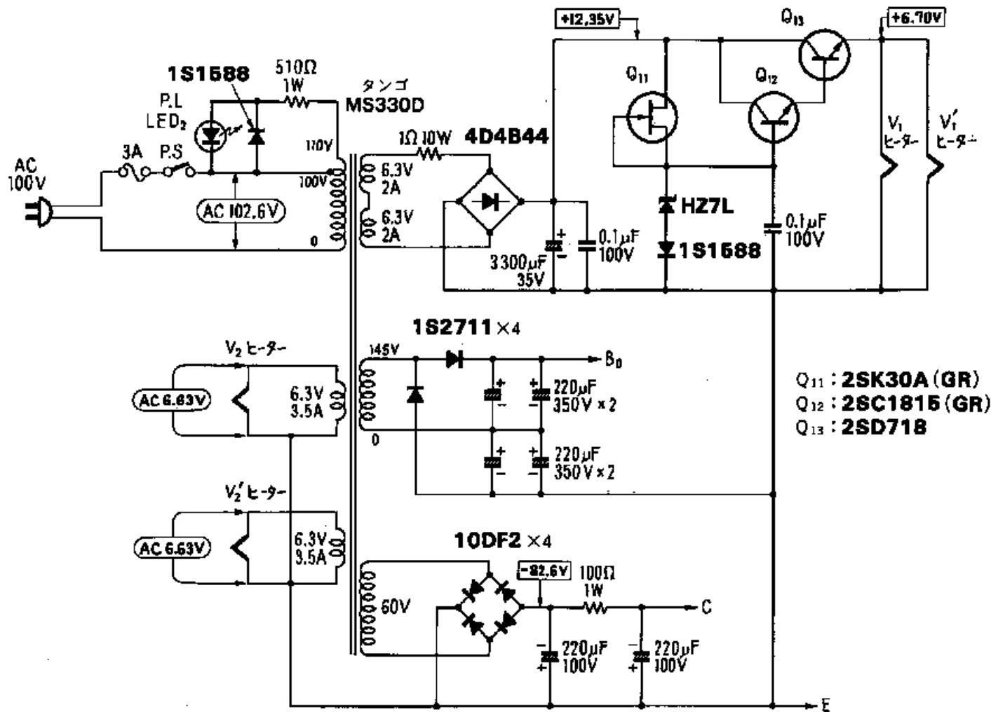
【図 13】 電源部回路図 (両 ch 分)
