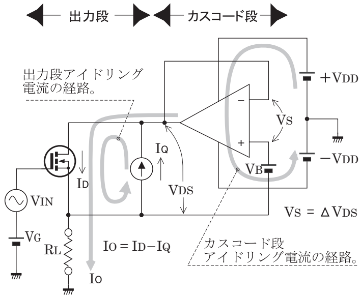
[ 図 7 ] B級プッシュプルカスコード/ A級シングルソースフォロワ回路
