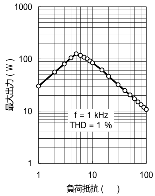
[ 图15 ] 负荷抵抗对最大出力特性
