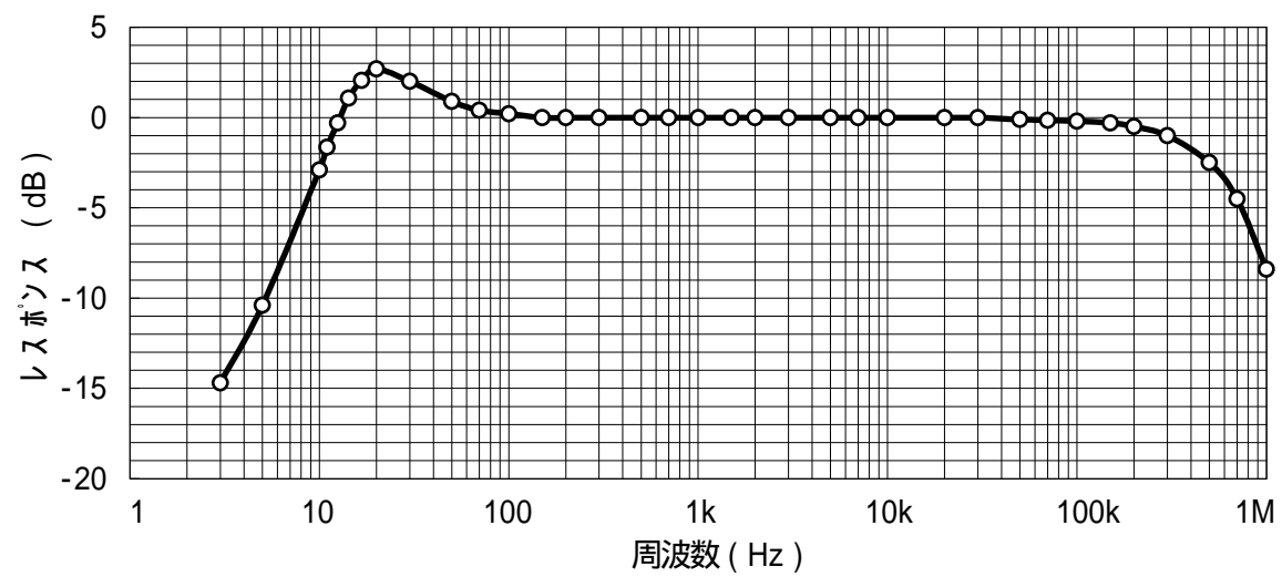
[ 図13 ] 周波数特性
