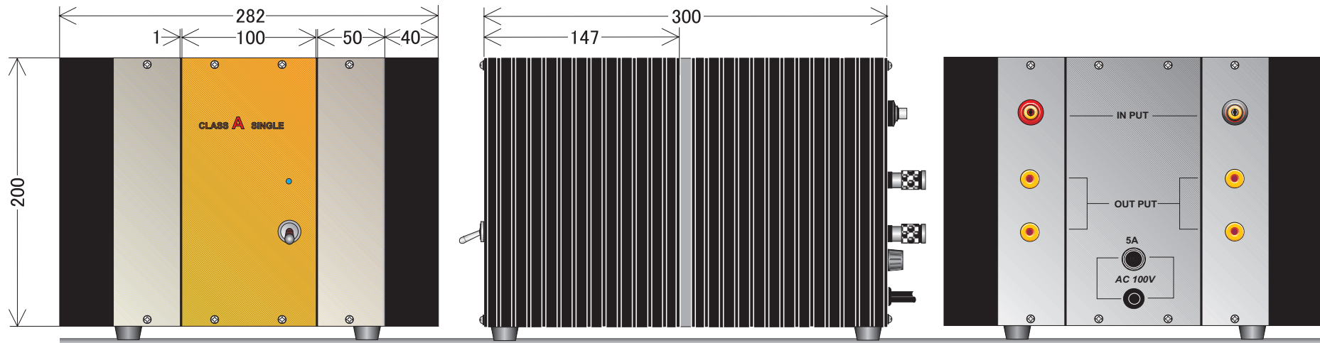
[ 図11 ] 外観と寸法
