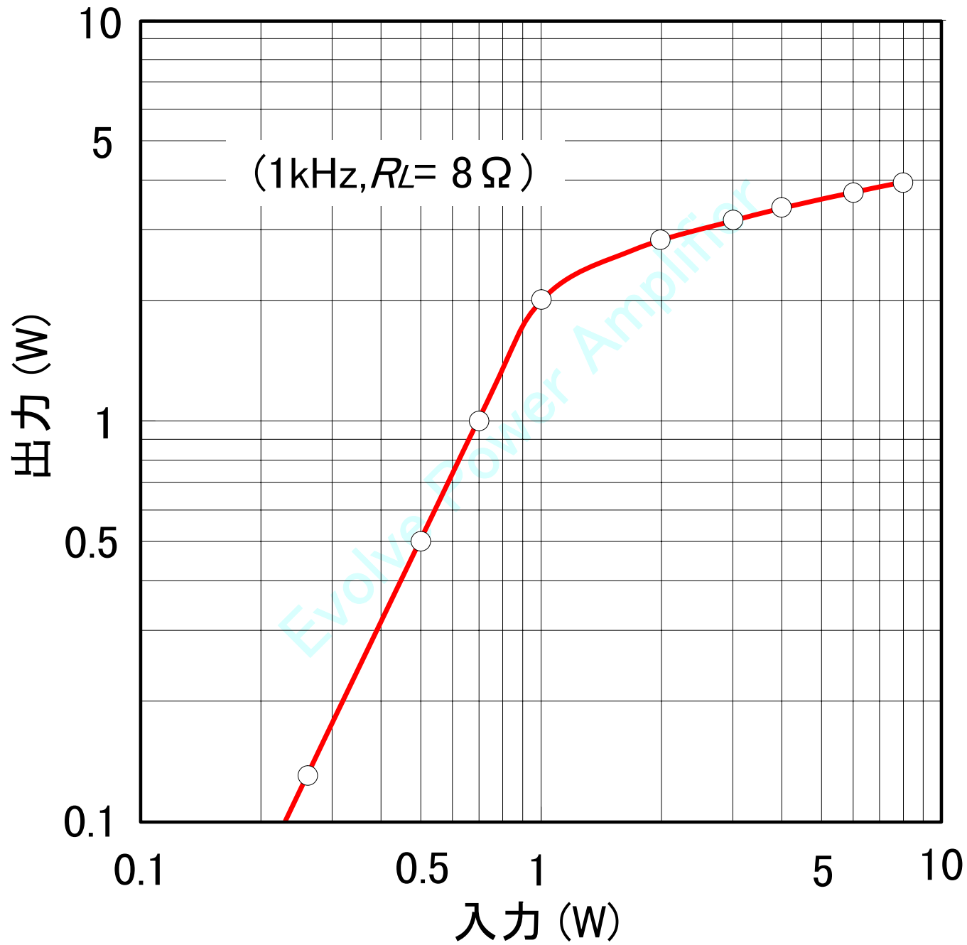
[図9] 入力対出力特性
