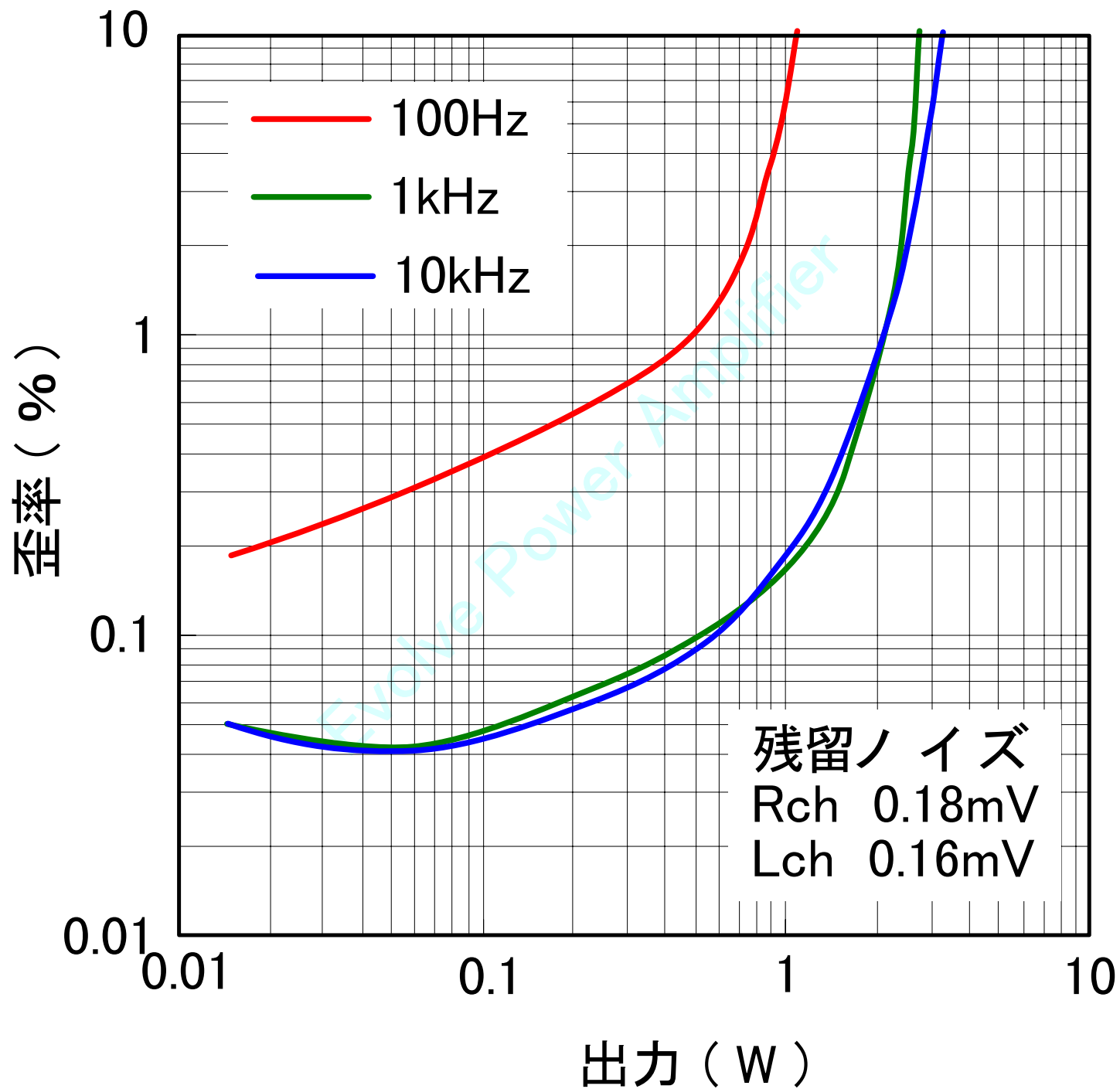
[ 図11 ] 出力対歪率特性
