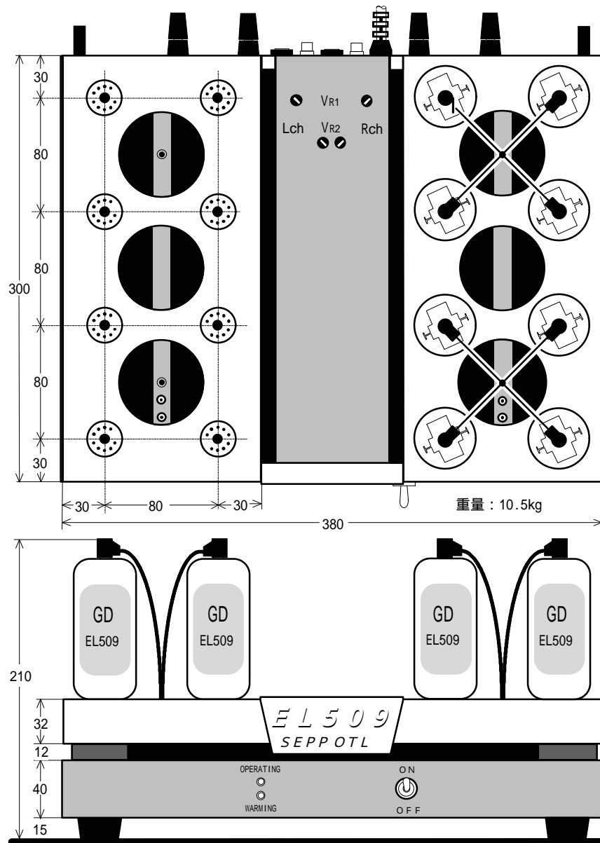
図 10 シャーシーのデザイン
