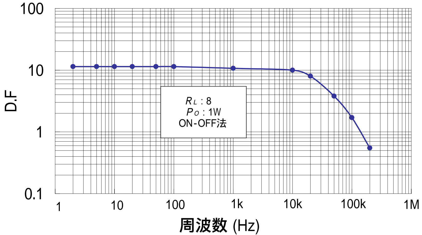
[ 図14 ] ダンピングファクタ-特性
