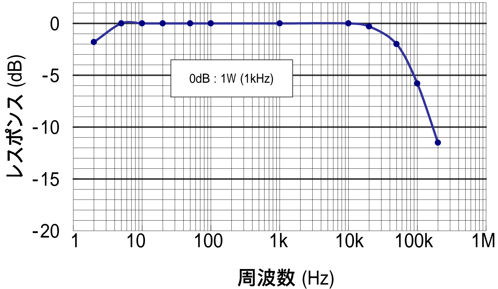
[ 図12 ] 周波数特性
