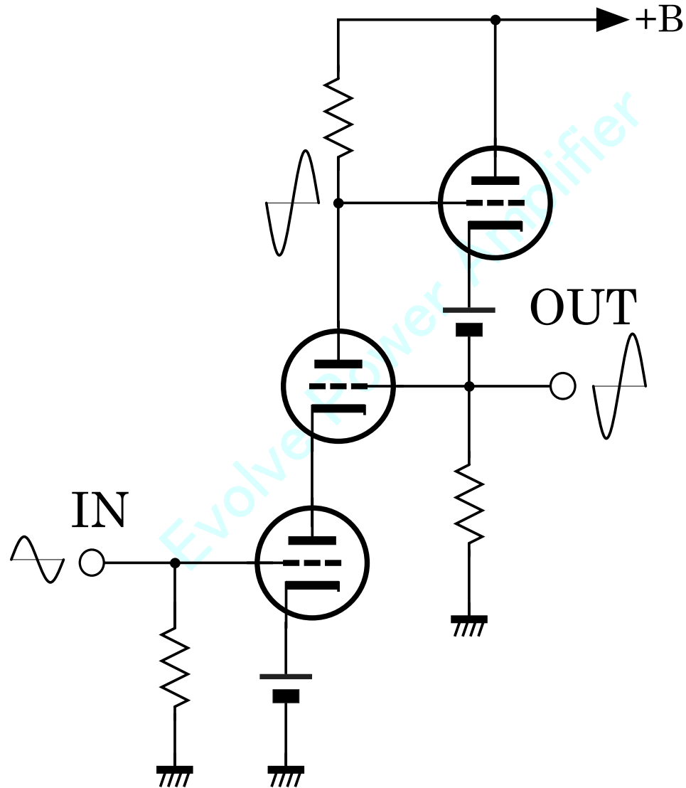
[ 図1 ] 超3結バージョン4 の基本回路
