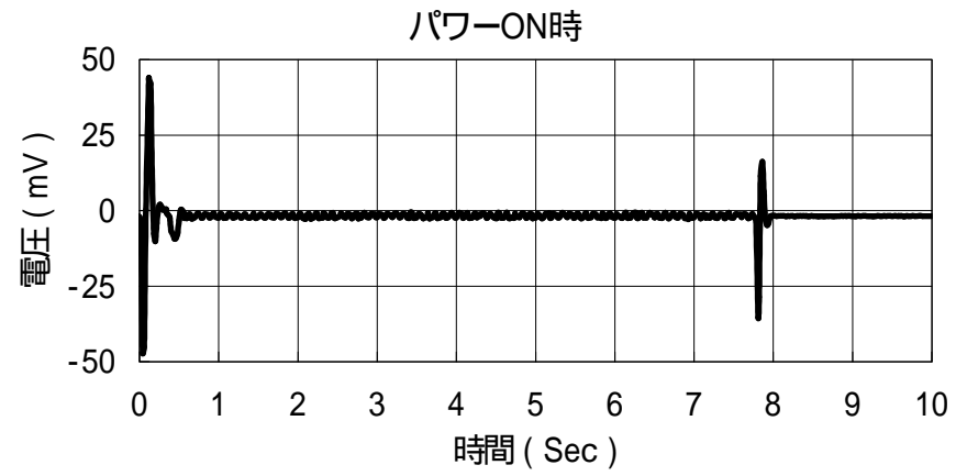
[ 図18 ] ショックノイズ波形
