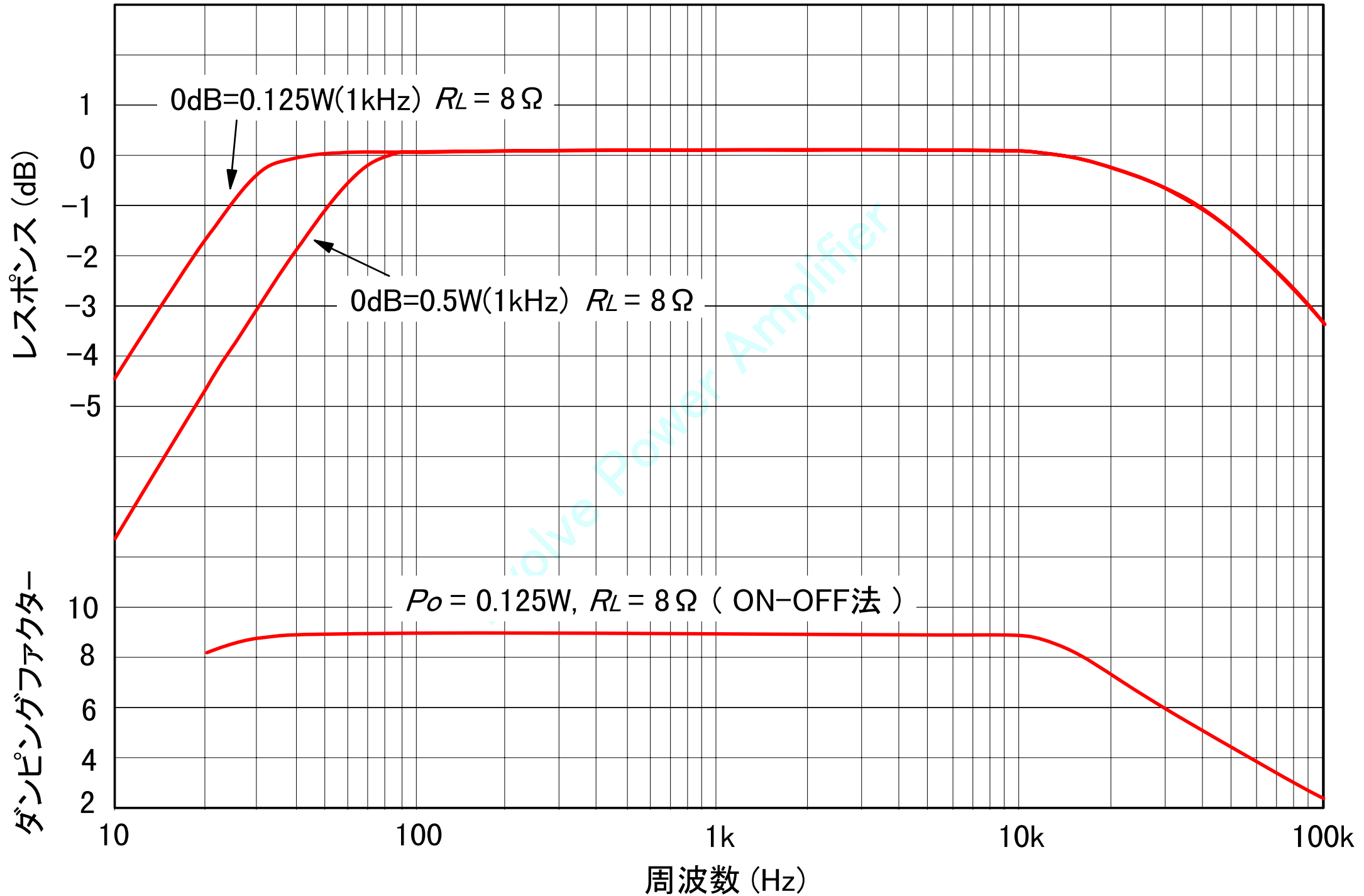
[ 図 10 ] 周波数特性とダンピングファクター特性
